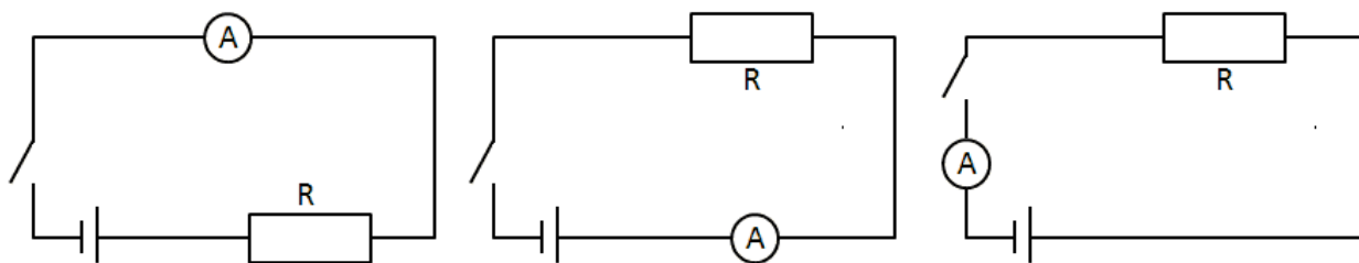
Рисунок 7.5. Исследуемые схемы для определения значений силы тока
