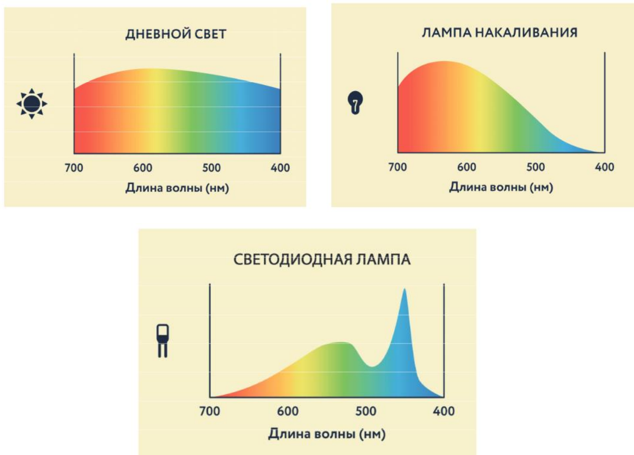
Рисунок 3.3. Спектр излучения для светодиода
