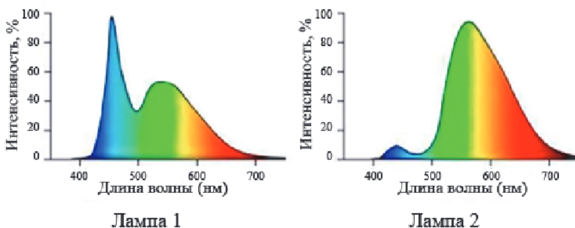
Рисунок 3.4. Зависимость интенсивности излучения от длины волны для светодиодных ламп
