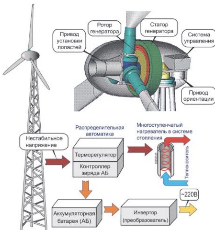
Рисунок 3.2. Принцип работы ветрогенератора
